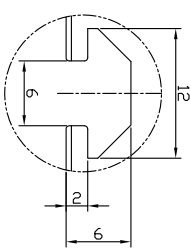
A部：スライドナット スロット
